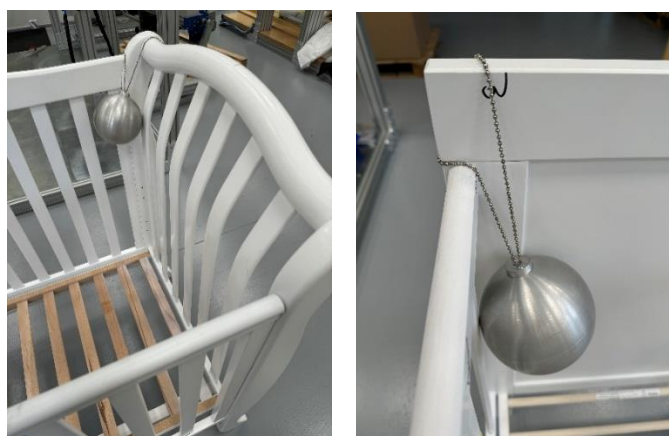
Obrázok č.3 – Skúšanie miesta zachytenia (simulujú možné zachytenie detského oblečenia na vonkajších a vnútorných stranách postelky)
