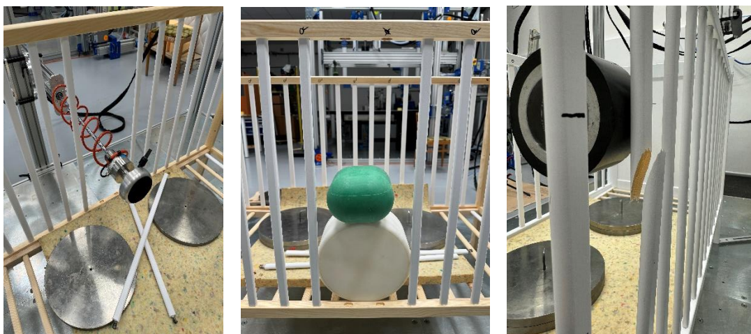
Obrázok č. 1 – Skúška pevnosti bočníc a čiel (Statické zaťaženie lamiel)
