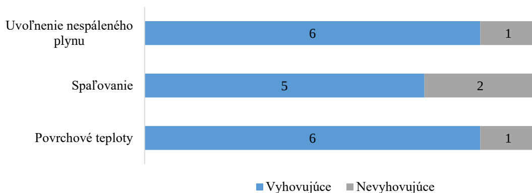
Graf č. 2 - Grafické znázornenie výsledkov testovania technických vlastností terasových ohrievačov
